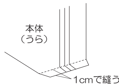
〈図1〉 マチの縫い方
